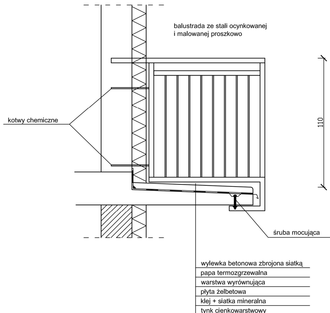
Szkic poglądowy balustrady balkonowej.
